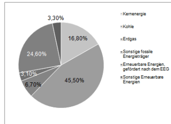
Stromerzeugung 2012 in Deutschland - Durchschnittswerte
